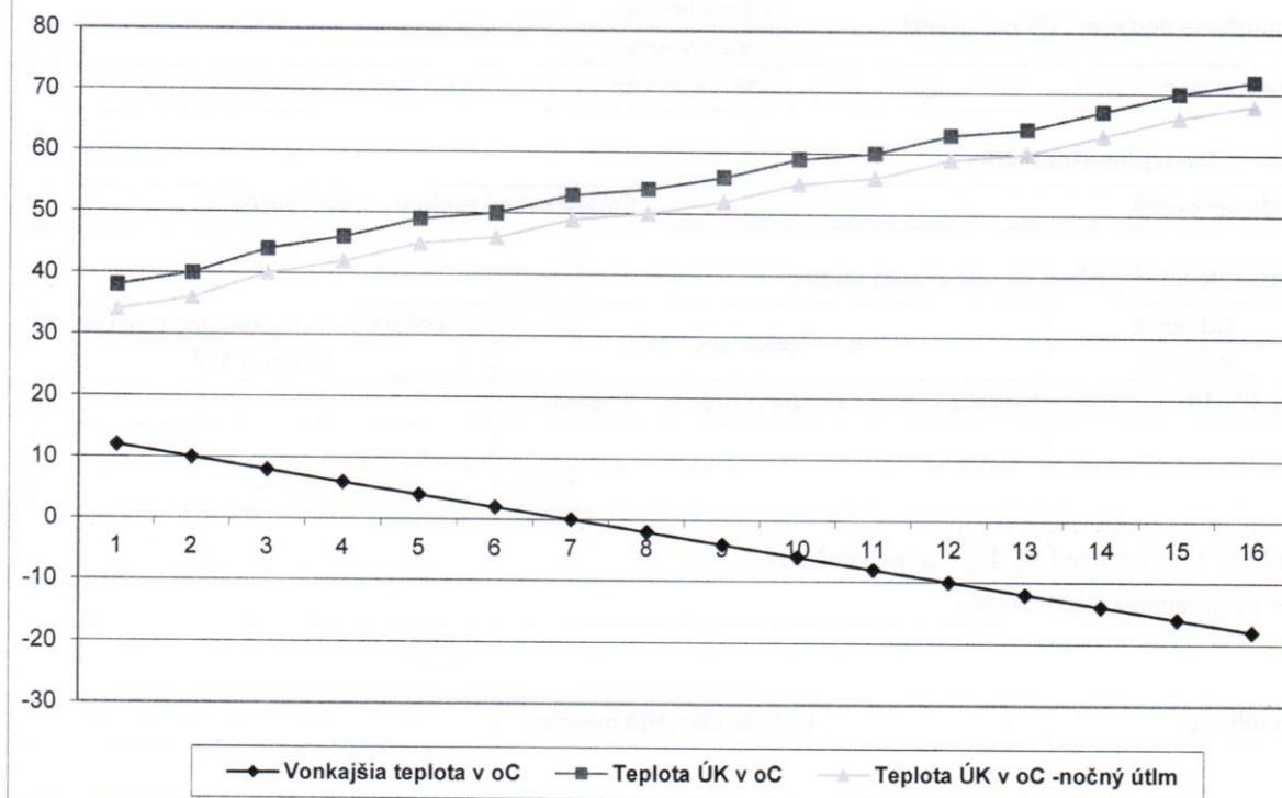
Vykurovacía tabuľka ÚK podľa vonkajších teplôt
